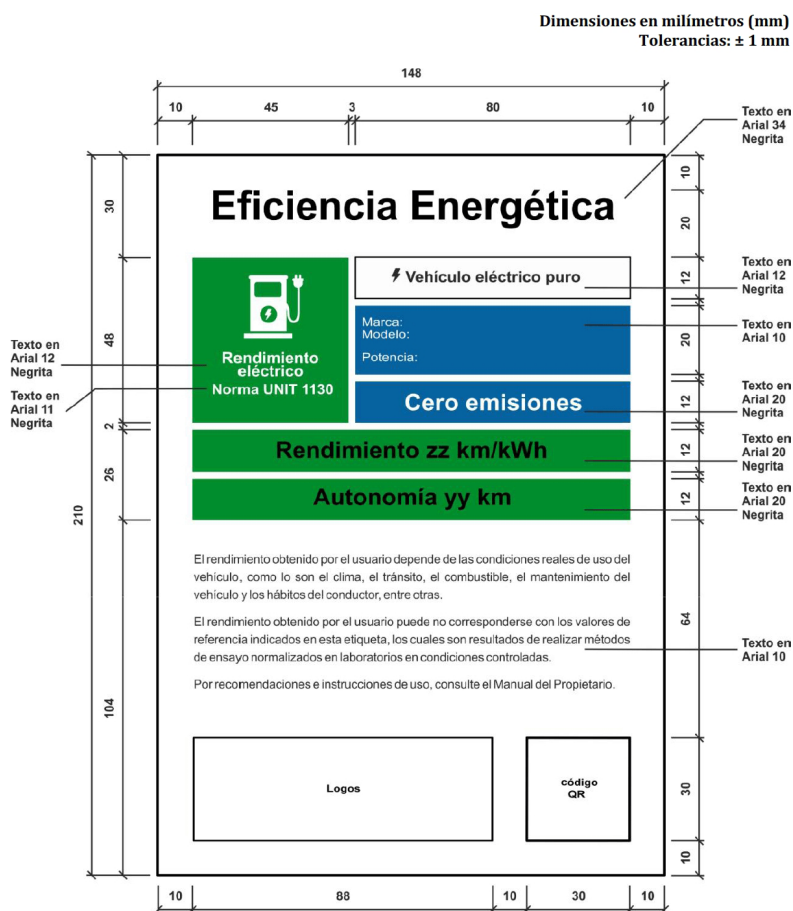
Figura 7. Etiqueta para vehículos eléctricos puros prevista na Norma UNIT 1130:2020.
