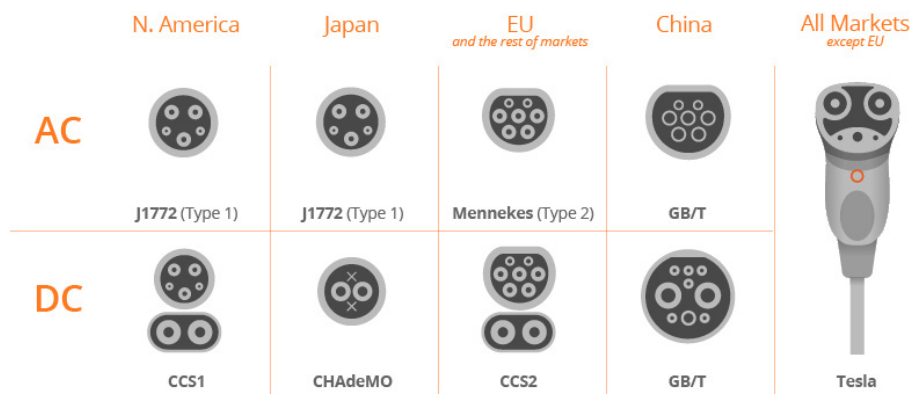
Figura 2. Padrões de conectores predominantes nos mercados globais atualmente.
