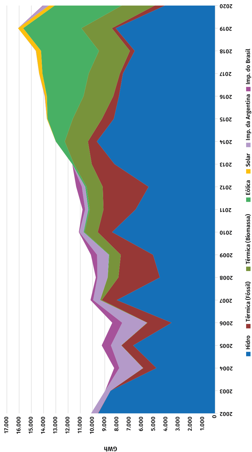
Figura 5. Geração de eletricidade por fonte e importação por país de origem.
