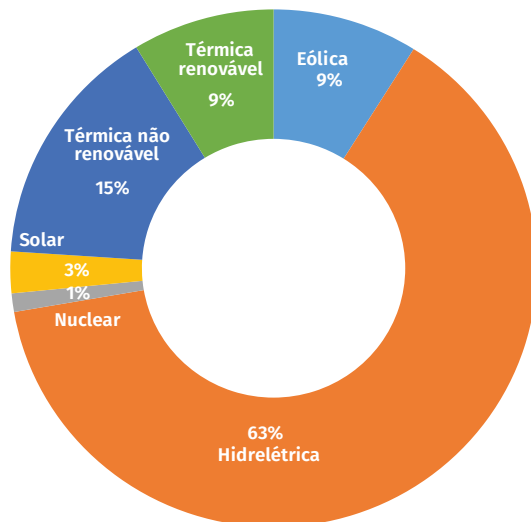
Figura 2. Capacidade instalada por fonte 2019.
