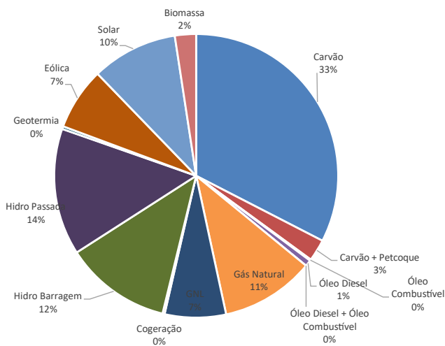
Figura 9. Geração SEN em % por fonte 2020, 77.696 GWh. Fonte: CNE.
