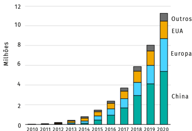
Figura 1. Evolução do estoque de veículos elétricos (2010-2020)
