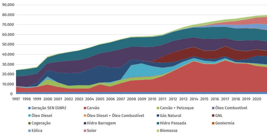
Figura 8. Geração SIC + SING e SEN por combustível, 1996-2020 GWh. Fonte: CNE, GWh.
