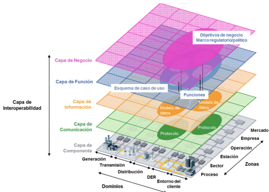
Figura 1. Modelo de Arquitetura de Smart Grid (SGAM).
