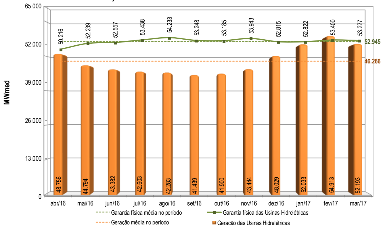
Figura 23. Acompanhamento da geração verificada e da garantia física das usinas hidrelétricas (UHE, PCH e CGH).
