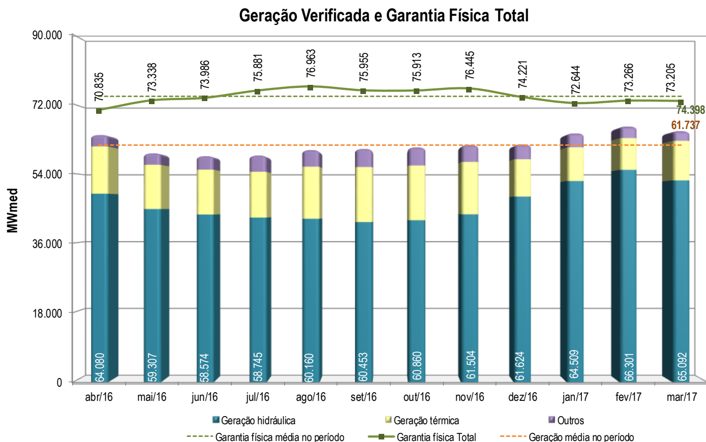
Figura 29. Acompanhamento da geração verificada e da garantia física das usinas do SIN.
