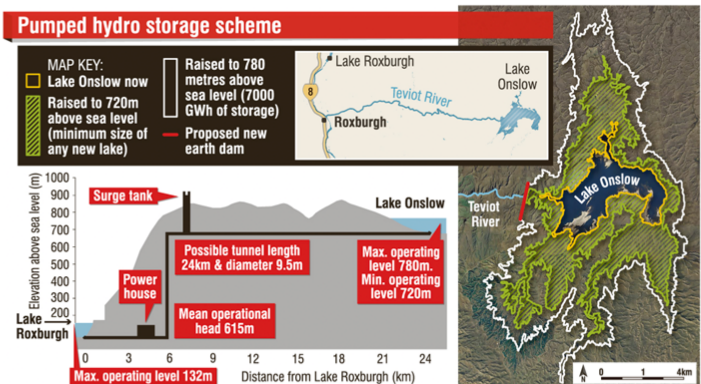
Figura 2 Projeto da UHR de Lake Onslow.
