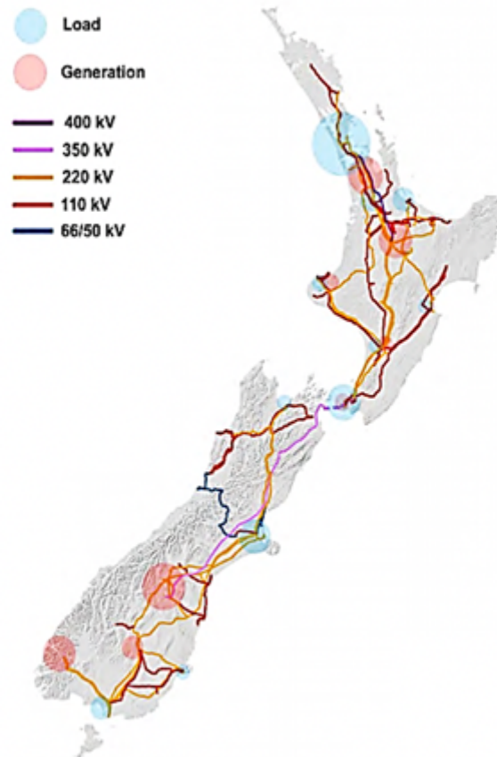
Figura 1 O sistema de Transmissão da Nova Zelândia: 2018.
